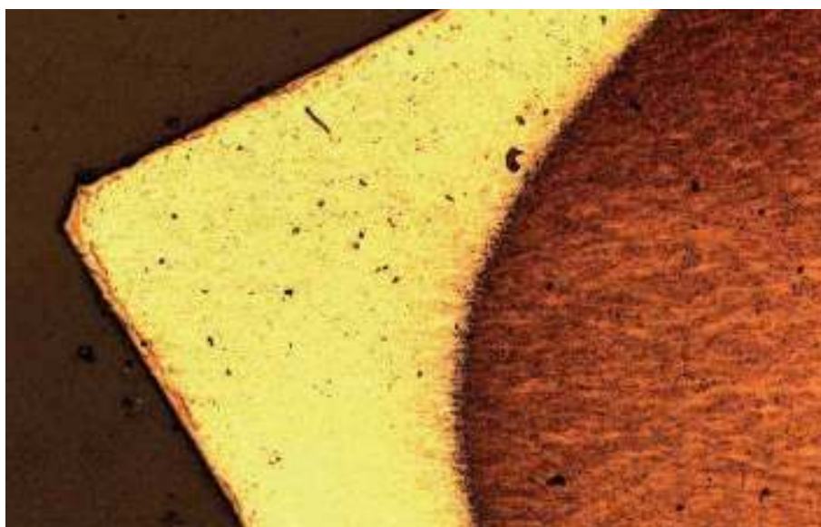
Primer plano de un filo de corte tras el templeado por inducción. La parte del filo con templeado especial (claro) destaca de forma precisa la microestructura más blanda del cuerpo del alicate (oscuro).
