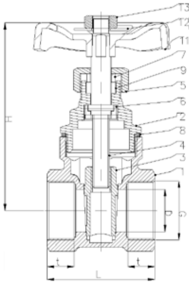
DN15 - DN25
