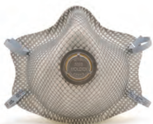
2310 N99
