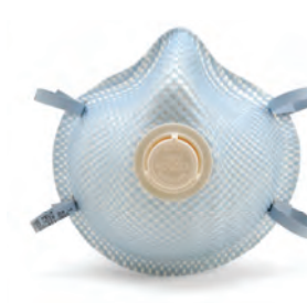
▲ 2300N95
