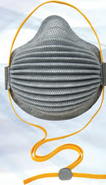
● 4800 N95
