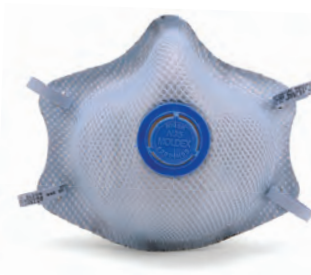
■ 2500N95
